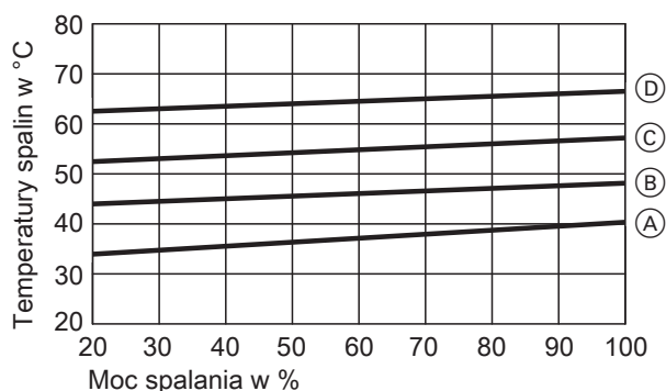
Temperatura spalin kotła Vitocrossal, typ CRU, 800 kW
